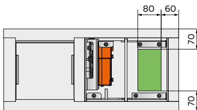
Bereich für Bohrpositionen in fester Rückwand
