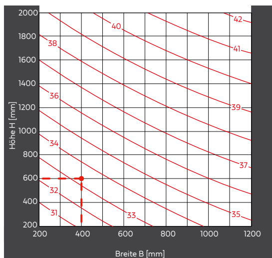
Schallleistungspegel L_{WA} [dB(A)] bei v = 5 m/s
