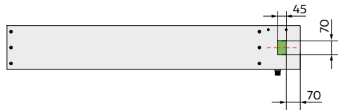
Bereich für Bohrpositionen von oben / unten
