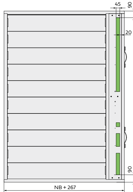
Bereich für Bohrpositionen von vorne
