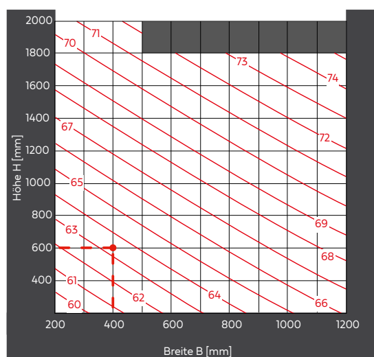
Schallleistungspegel L_{WA} [dB(A)] bei v = 15 m/s
