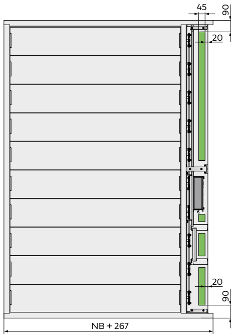
Bereich für Bohrpositionen in fester Rückwand
