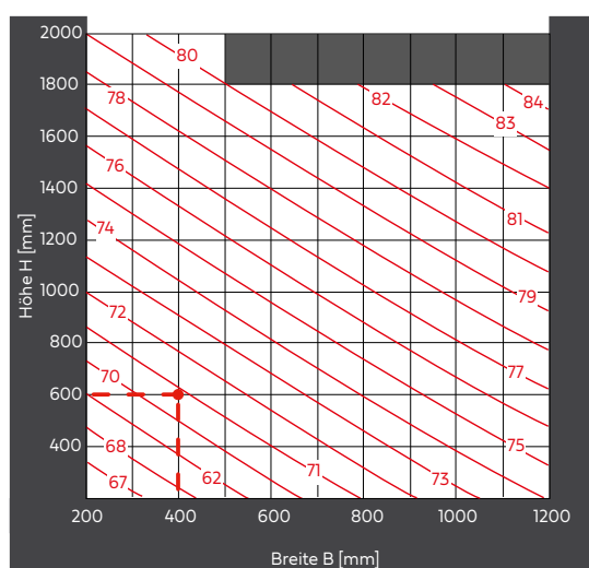
Schallleistungspegel L_{WA} [dB(A)] bei v = 20 m/s
