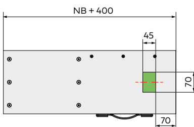
Bereich für Bohrpositionen oben / unten
