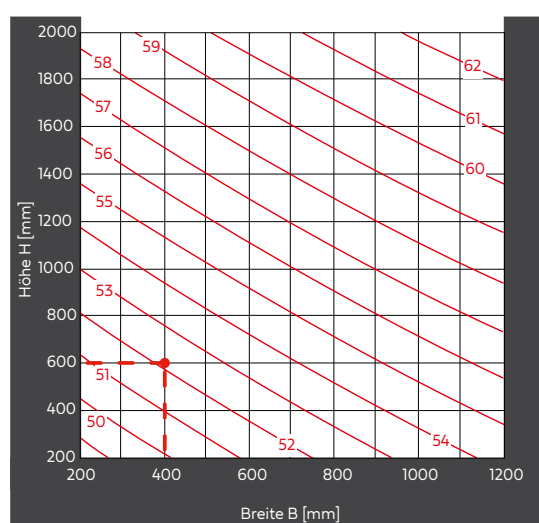
Schallleistungspegel L_{WA} [dB(A)] bei v = 10 m/s
